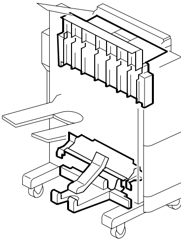
4. EXTERIOR 4 (B546)
