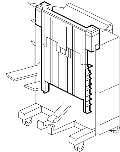
3. EXTERIOR 3 (B546)
